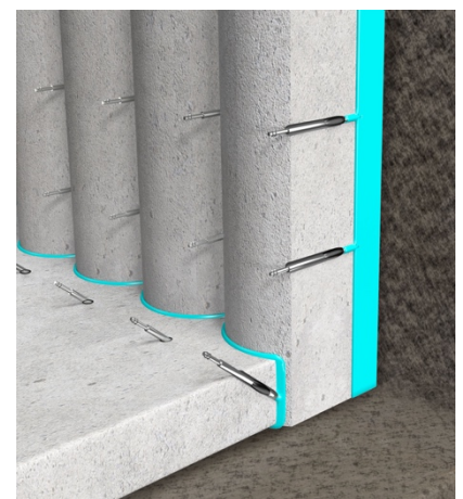
Uszczelnienie palościanki
